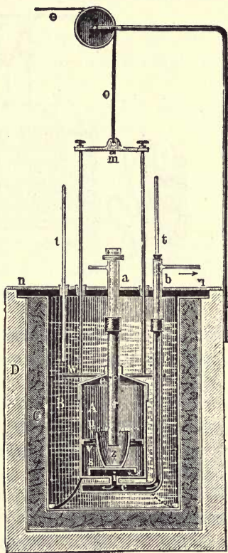
FIG. 25. — Fischer's Calorimeter.
