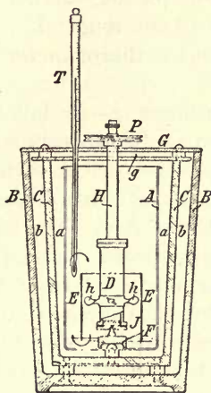
FIG. 27. — Parr Calorimeter.
