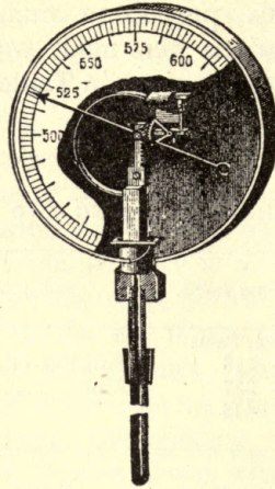
FIG. 6. — Thalpotasimeter (Klinghammer).
