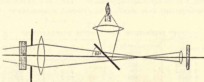
FIG. 16. — Optical Pyrometer (Cornu-Le Chatelier).
