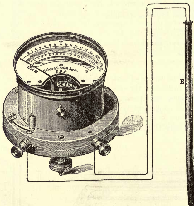
FIG. 22. — Holborn-Wien Pyrometer.
