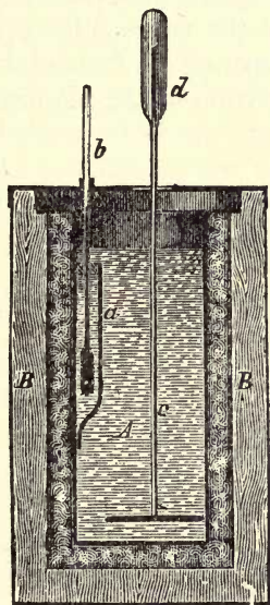
FIG. 12. — Fischers Calorimeter.
